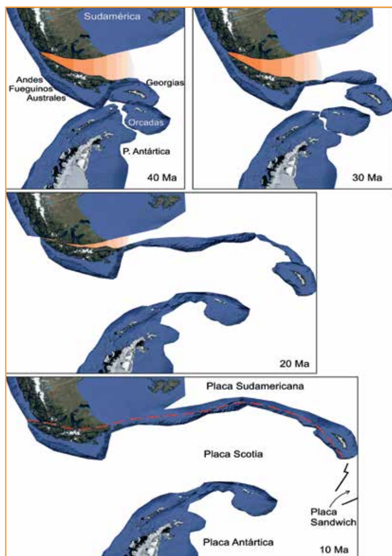
Figura 1. Modelo tectónico que muestra las posiciones teóricas de los fragmentos continentales que formaban la conexión Sudamérica-Antártida, desde hace 40 millones de años (Ma) hasta hace 10 Ma. A partir de entonces y hasta la actualidad, la línea roja se convirtió en el límite de las placas Sudamericana (al norte) y de Scotia (al sur).
